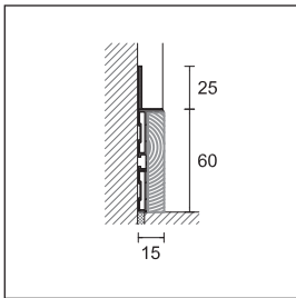
88/6 + 88/16SF inserção em madeira
