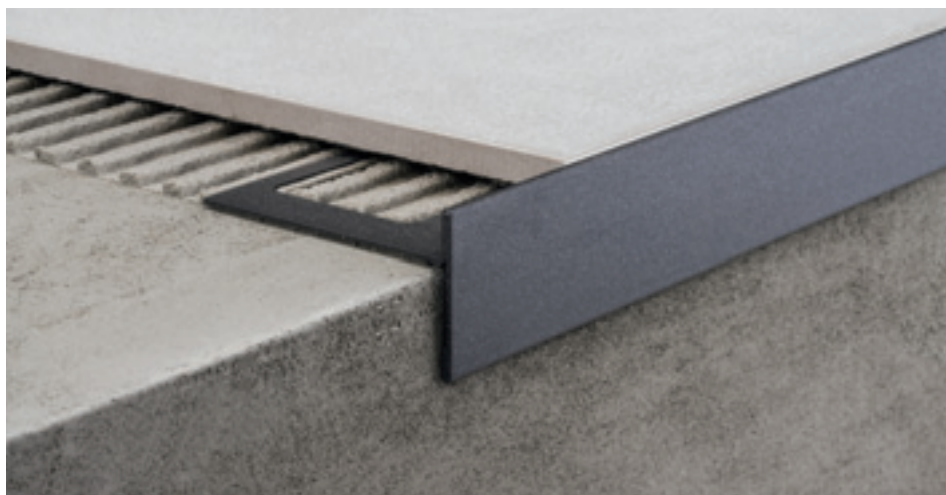
CPEV/45/12 alumínio lacado cinza antigo
