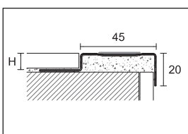
SIX/10 aço inox escovado AISI 304 - DIN 1.4301 + antiderrapantes preto 25 mm
