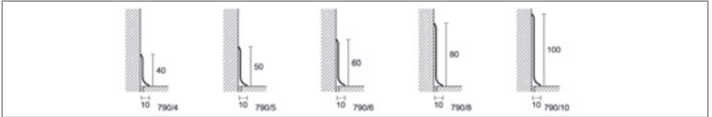
790/6 aço inox polido AISI 304 DIN 1.4301
