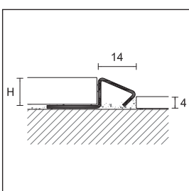
MIN/10 aplicação para pisos de altura diferente
