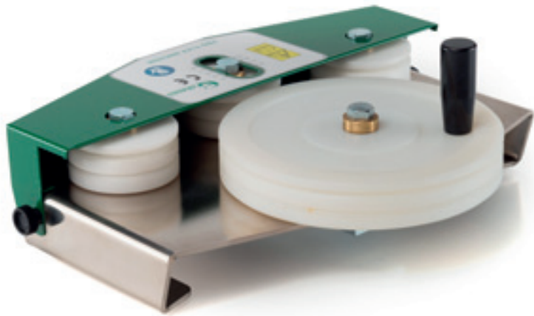
PROFLEX MACHINE - máquina manual para curvar os perfis proflex line
