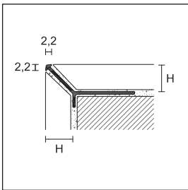
IPA/11 alumínio anodizado prata
