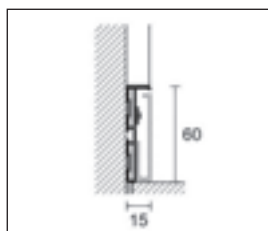
87/6 + 88/16L/A inserção em alumínio para LED
