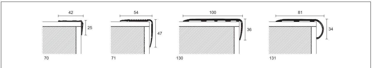
71/SF alumínio anodizado prata
