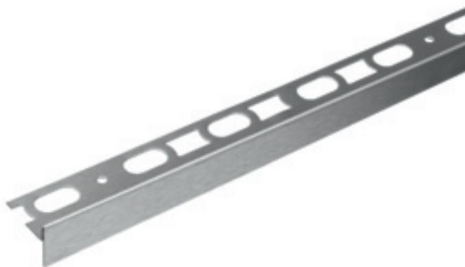
GPS3/DX/10 aço inox escovado AISI 304 DIN 1.4301
