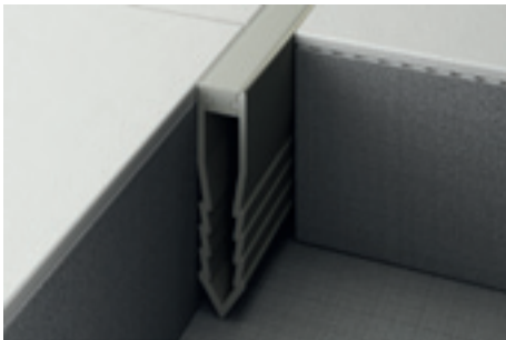
NF/45 PVC coextrudido cinza + cinza RAL 7035
