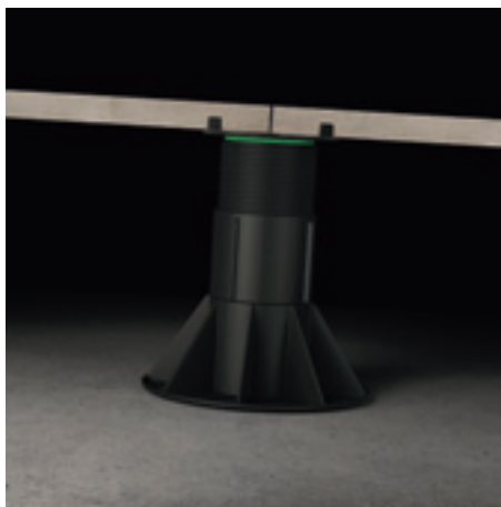
Com o anel conversor "Perfect Ring" inserido, o suporte fica fixo.
