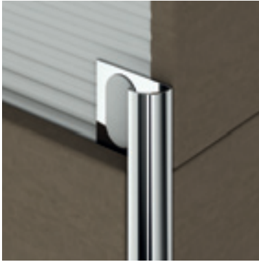
RKN/10 latão cromado
