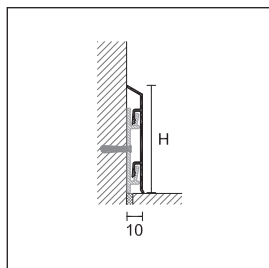
95/7 alumínio anodizado prata
