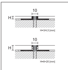
NTA/10 alumínio natural + EPDM cinza resistente ao polimento RAL 7046
