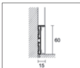
87/6 + 88/16SF inserção em alumínio
