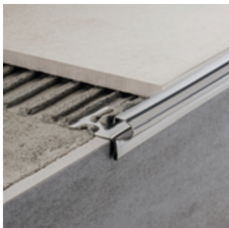
SGI/11 aço inox polido AISI 304 DIN 1.4301
