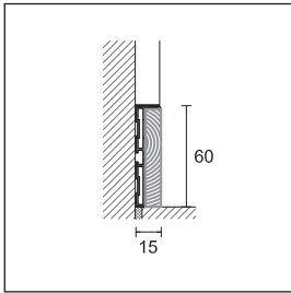
87/6 + 88/16SF inserção em madeira
