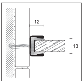
GPS14/12 aço inox escovado AISI 304 DIN 1.4301
