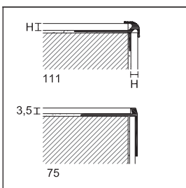
111/4/F alumínio anodizado prata
