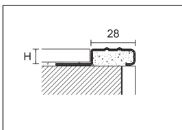
SIS/10 aço inox escovado AISI 304 - DIN 1.4301
