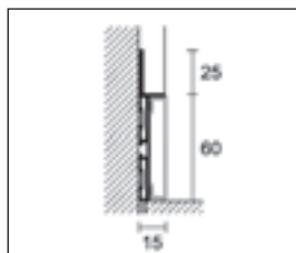
88/6 + 88/16SF inserção em alumínio
