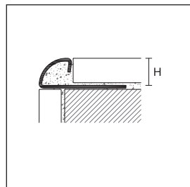
RIL/10 aço inox AISI 304 DIN 1.4301
