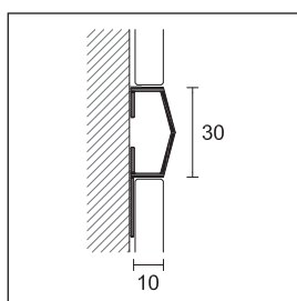
AVK/1 latão cromado
