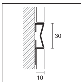
AVK/2 latão cromado
