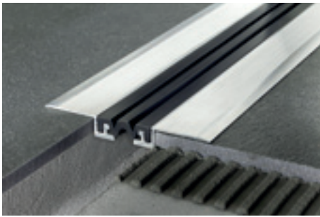
GJF/40 alumínio natural + EPDM preto RAL 9005
