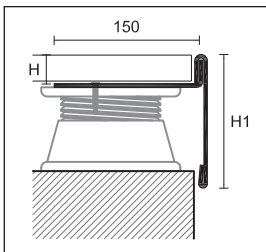
CPLB + CPLV/60 alumínio lacado cinza claro RAL 7038
