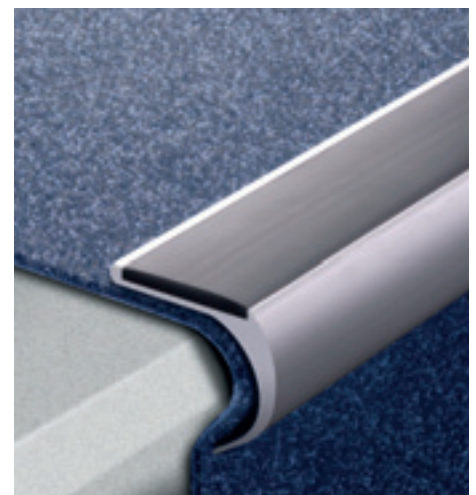
128/F alumínio anodizado prata
