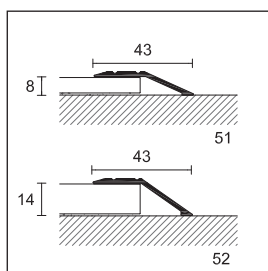
51/A alumínio anodizado ouro
