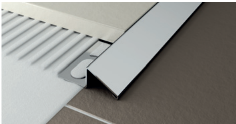
PNI/10 aço inox polido AISI 304 DIN 1.4301
