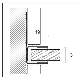
GPS2/19 aço inox escovado AISI 304 DIN 1.4301
