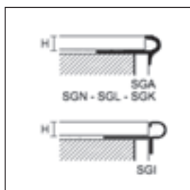
SGI/11 aço inox polido AISI 304 DIN 1.4301
