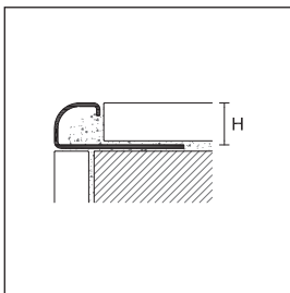
RIN/10 aço inox AISI 304 - DIN 1.4301
