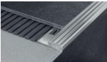
SIS/10 aço inox escovado AISI 304 - DIN 1.4301
