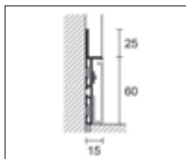
88/6 + 88/16L/A inserção em alumínio para LED
