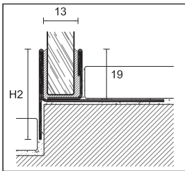
GPS1/DX/19 aço inox escovado AISI 304 DIN 1.4301
