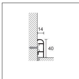
97/4TMSF alumínio brilhante escovado titânio
