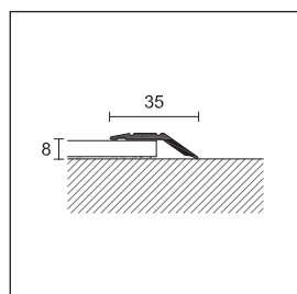
355/A latão polido
