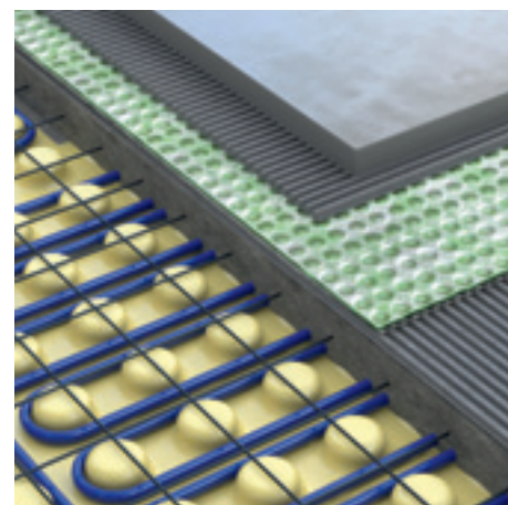
PWP30 - pavimento radiante
