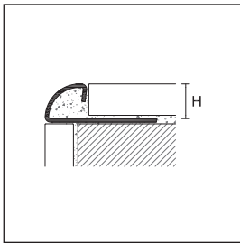
RKN/10 latão cromado
