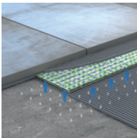
PWP30 - escoamento do vapor
