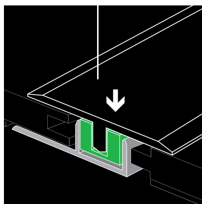
presionar el perfil superior contra la base
