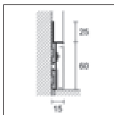
88/6 + 88/16L/A inserción en aluminio para LED
