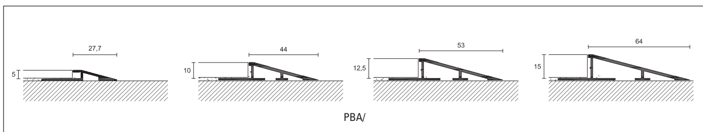
PBA/10 aluminio anodizado plata
