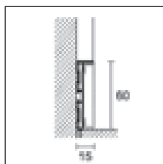
87/6 + 88/16SF inserción en aluminio
