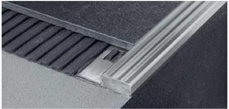
SIS/10 acero inoxidable satinado AISI 304 - DIN 1.4301
