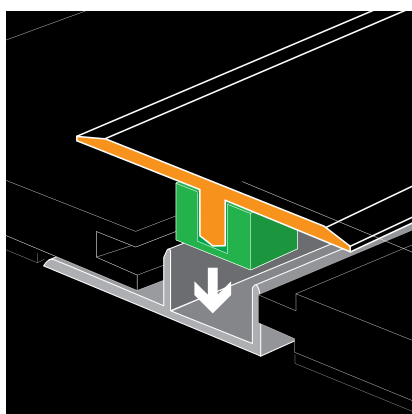
poner el perfil superior en la base
