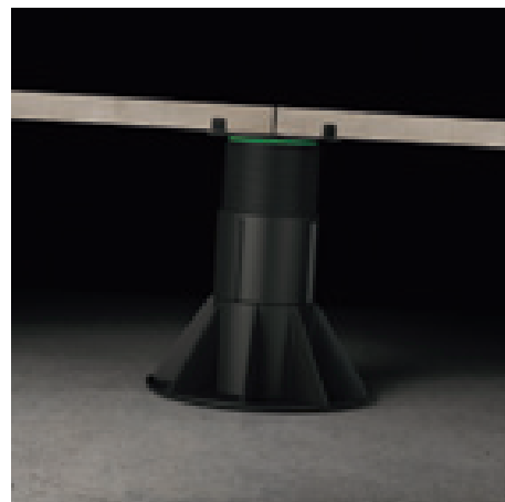
con el anillo convertidor Perfect Ring insertado, el soporte es fijo
