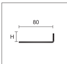
CPLB/2 base tallada para pavimento cerámico
