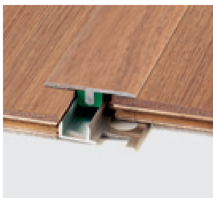
Z/1/SF aluminio revestido Alchrom® Plus
