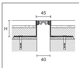
PBE/40 goma estriada
