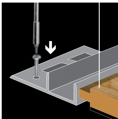
fije la base de aluminio al suelo con tornillos o pegamento
