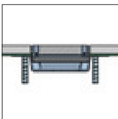
Classic Cover alicatado con el mismo pavimento.
