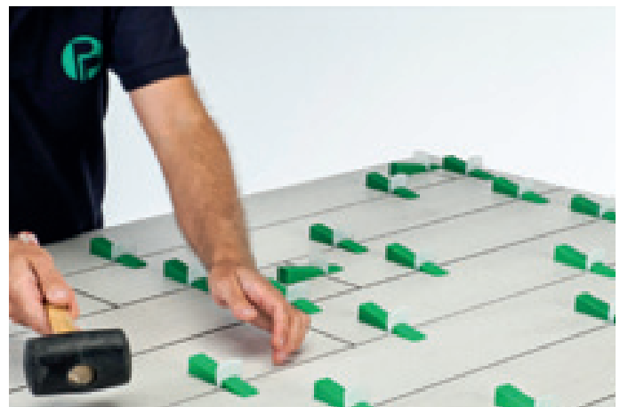
eliminación junta y cuña
