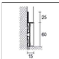
88/6 + 88/16SF inserción en aluminio
