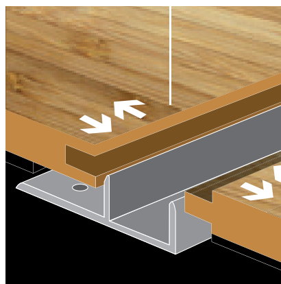
acercas las lamas del pavimento
