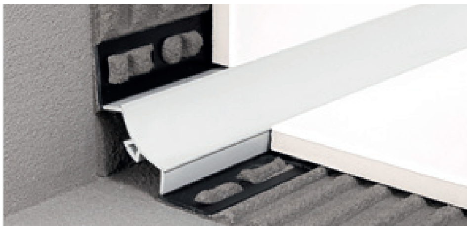
GP/10 PVC coextruido blanco
