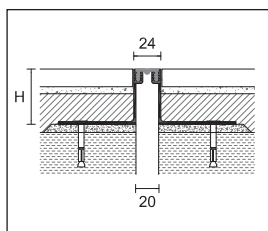
PBE/20 goma lisa
