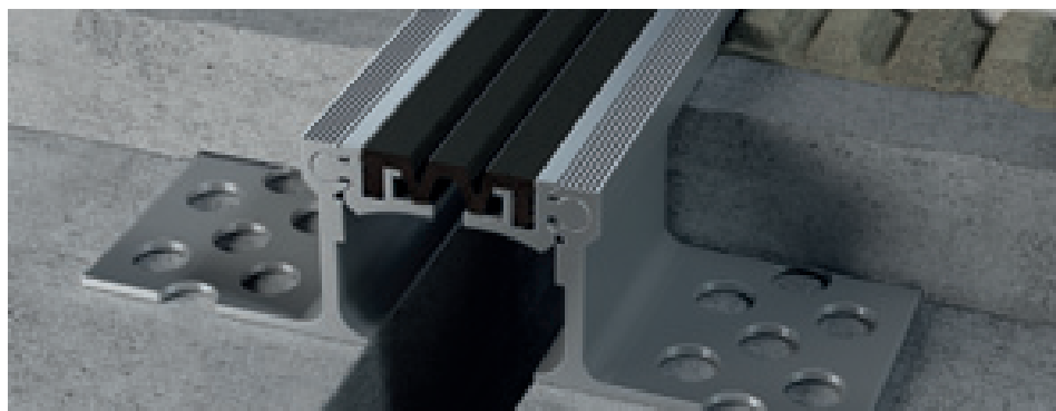
PBH/65/ aluminio natural + inserto EPDM negro
