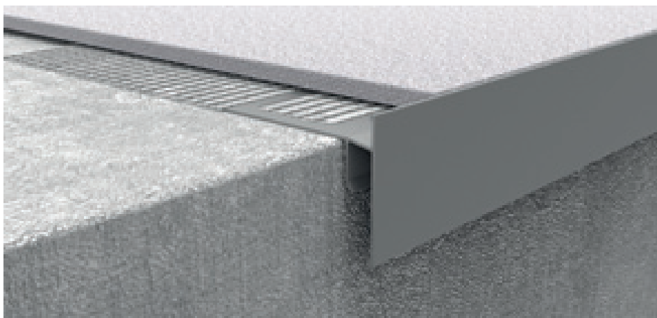
CPQV/50/10 aluminio lacado gris ceniza RAL 7038 arrugado
