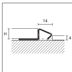
MIN/10 aplicación para pavimentos a distinto nivel
