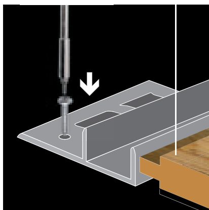
fissare la base in alluminio al sottofondo con viti o colla
