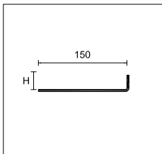
CPLB base per pavimenti sopraelevati
